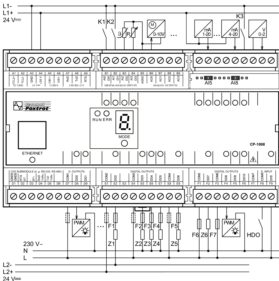
Obr. 4.1 Příklad zapojení binárních a analogových vstupů/výstupů základního modulu CP-1008
