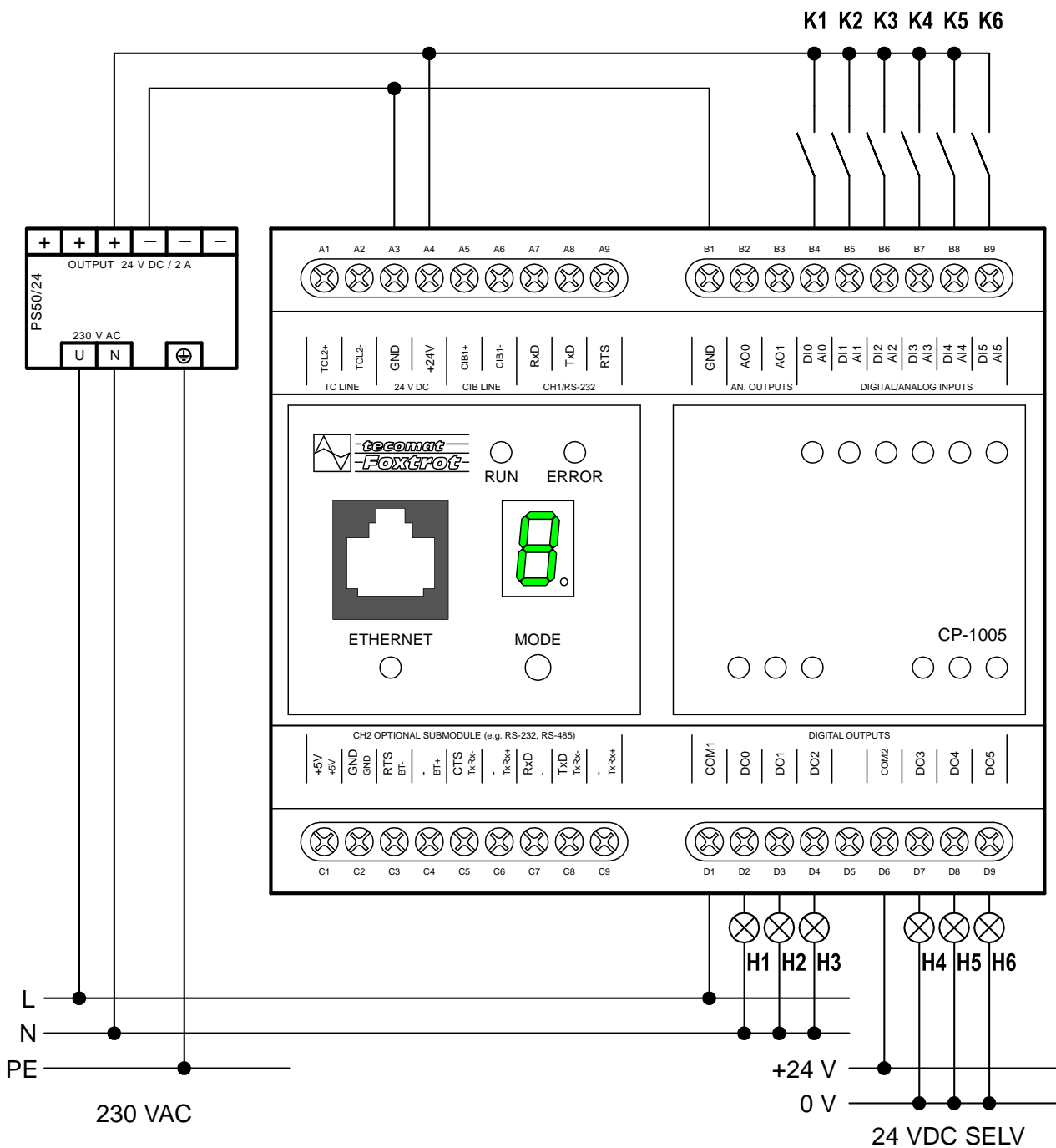
Obr. 4.1 Základní zapojení modulu CP-1005
