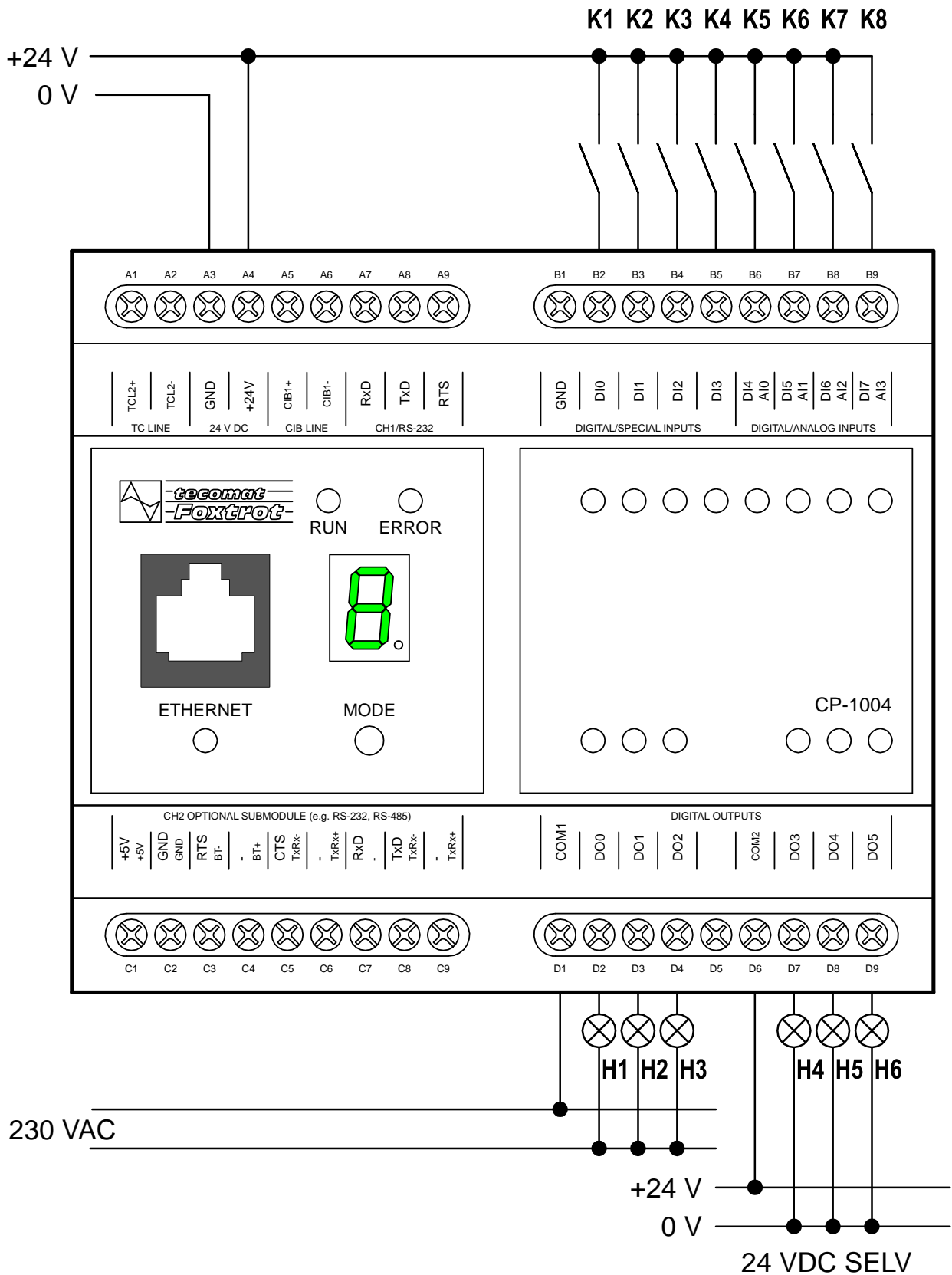
Obr. 5.1 základní zapojení modulu CP-1004
