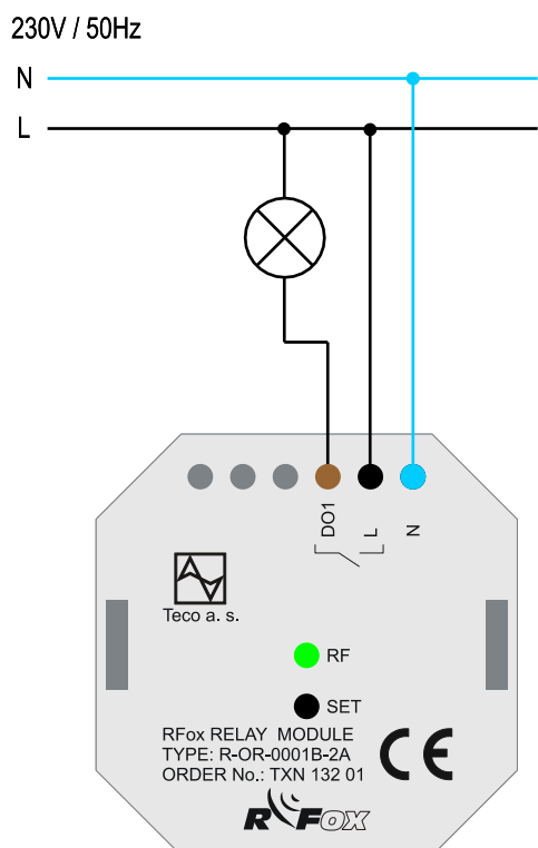
Obr. 3.13 Příklad zapojení
